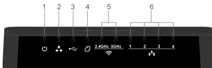
Рисунок 2 – Внешний вид передней панели RG-35-WZ
